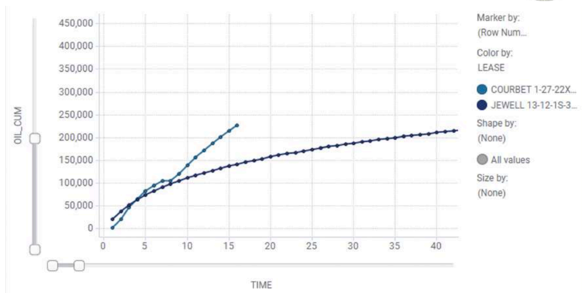
Abbildung 6: Kumulative Ölproduktion des Courbet-Bohrlochs bis dato (Barrel Öl) über Zeit (Monat) im Vergleich zu der Ölproduktion des Jewell-Bohrlochs. Brookside war sehr konservativ mit seiner geschätzten Produktion für das Jewell-Bohrloch, das aus der Woodford-Formation produziert.
