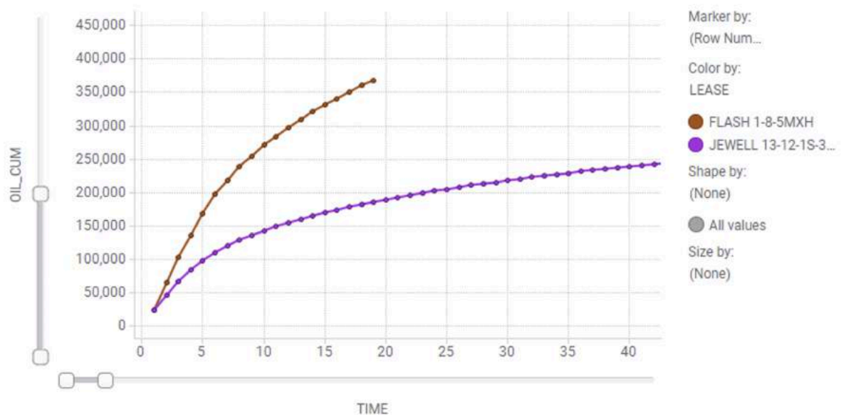
Abbildung 5: Kumulative Ölproduktion der Flash-Bohrung bis dato (Barrel Öl) über Zeit (Monat) im Vergleich zur Ölproduktion der Jewell-Bohrung. Brookside war sehr konservativ mit seiner geschätzten Produktion für das Jewell-Bohrloch, die aus der Sycamore-Formation produziert.
