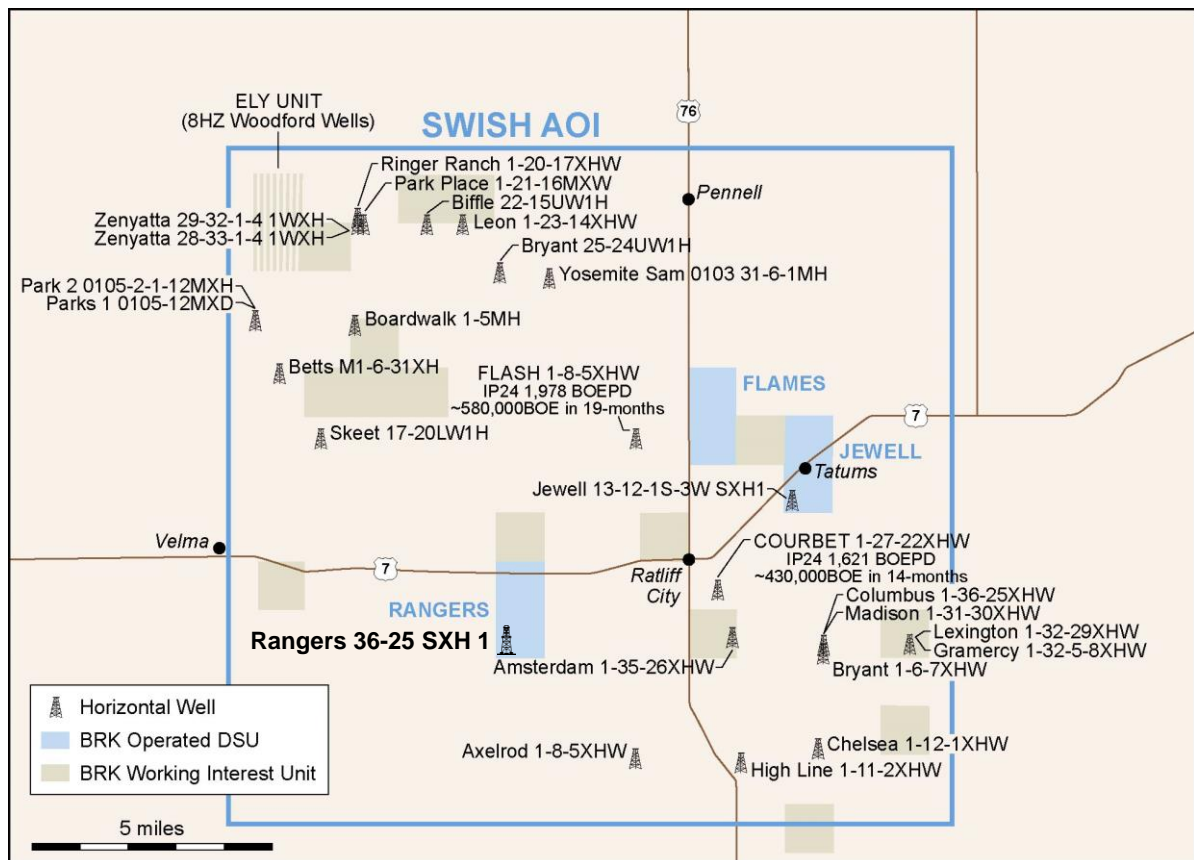
Abbildung 1: Lageplan mit dem Standort der Bohrung Rangers und den drei von Brookside bearbeiteten Erschließungszonen (DSUs) im Zielgebiet SWISH (AOI)
